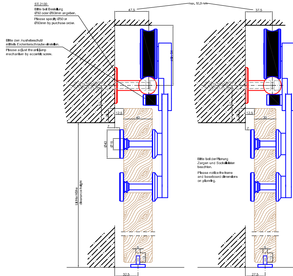
Beispiel mit 40mm Holztürblatt example with 40mm wooden door
