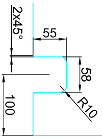
Glasausschnitt glass cut-out
