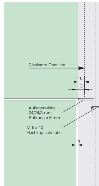
Ansicht Auflager - Oberlicht
