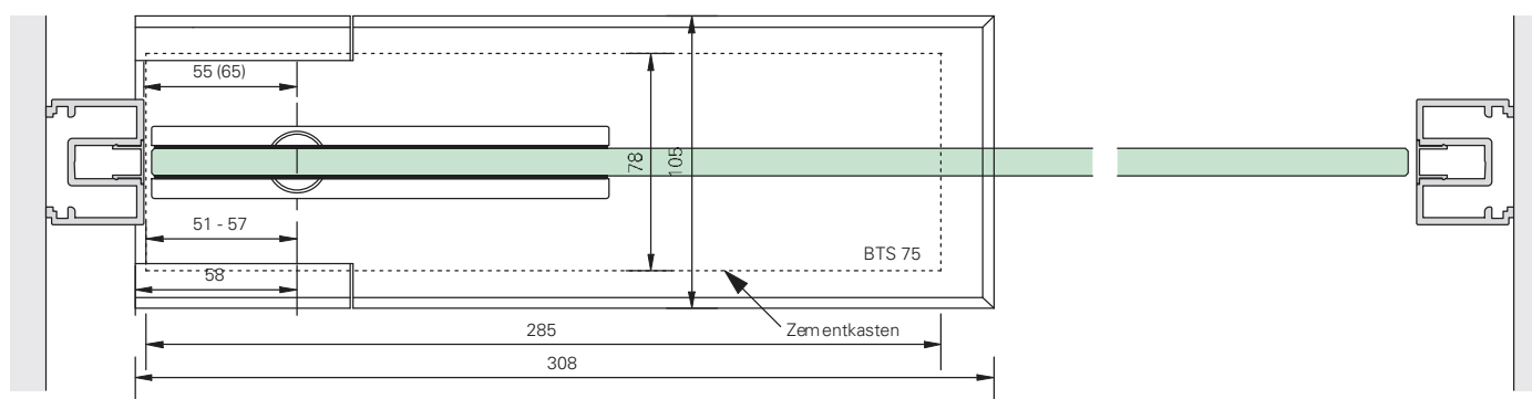
Grundriss / Pendeltür mit BTS 75
