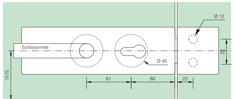
Ansicht Arcos Studioschloss mit Gegenkasten
