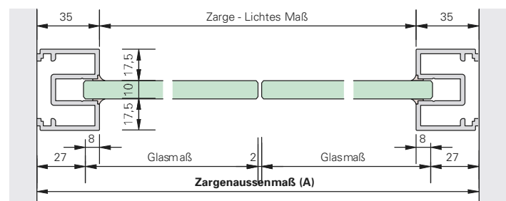
Festverglasung mit zwei Elementen
