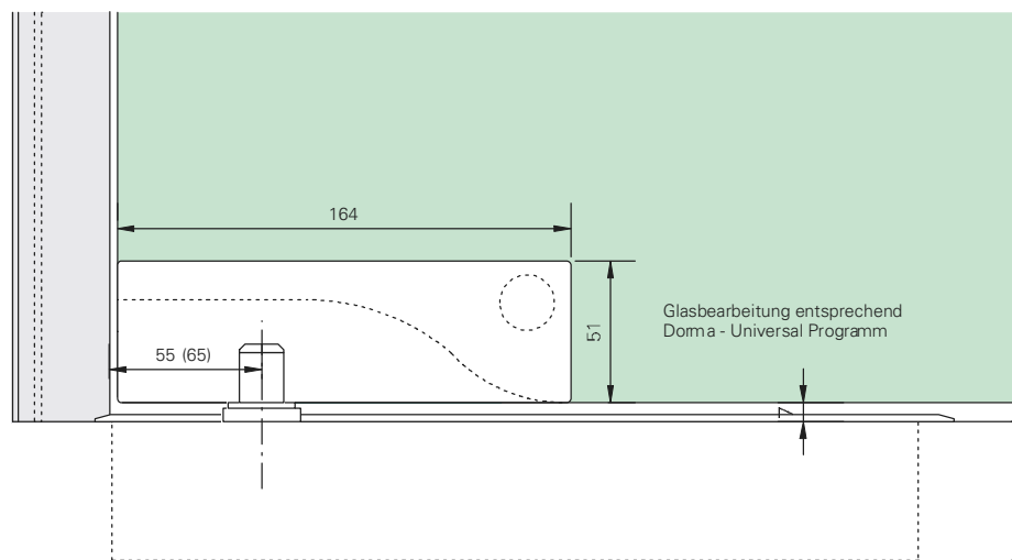
Ansicht Dorma Universal Band - Bodentürschliesser
