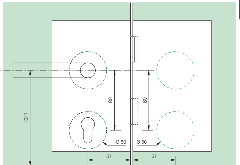
Ansicht Juniorschloss, Classic mit Gegenkasten
