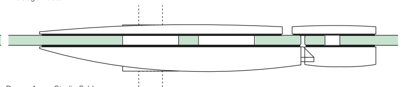
Dorma Arcos Studio Schloss
