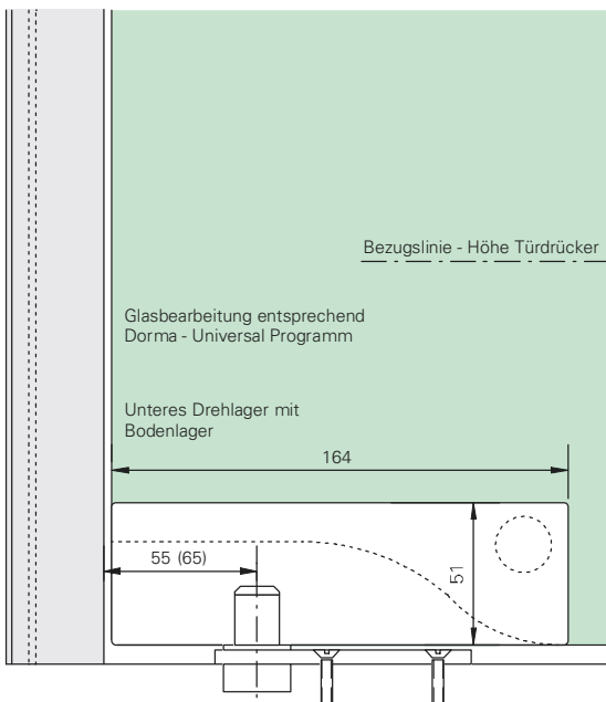
Dorma Universal Band unten
