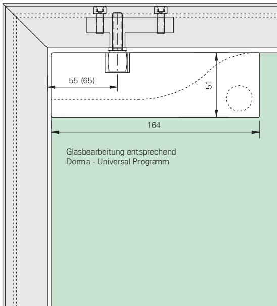
Ansicht Dorma Universal Band oben
