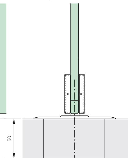
Schnitt - Bodentürschliesser
