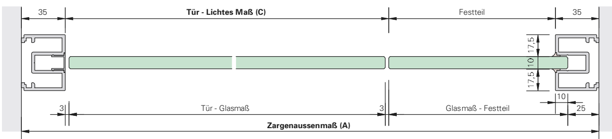
Tür mit Festverglasung
