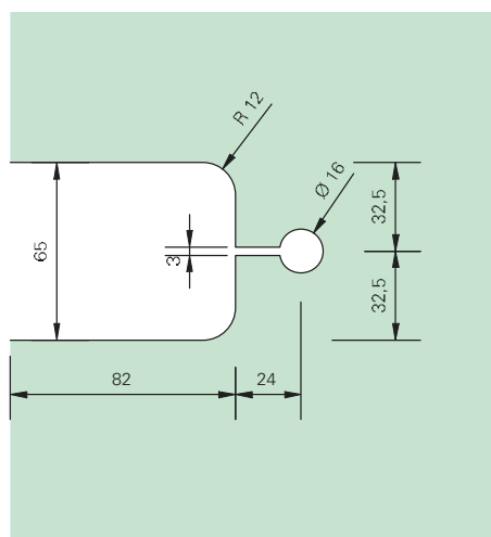
Glasbearbeitung Dorma - Tensor Programm
