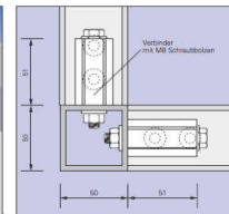
50.502 Eckverbindung Draufsicht
