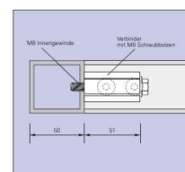
50.502 Stegverbindung Draufsicht
