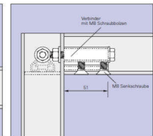
Schnitt senkrecht
